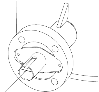
Рис. 7: Маркировочный паз.
